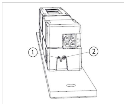
Obr. 5: Přehled řídicí jednotky ekey home RJE micro plus
