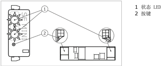
插图 6： ekey home 控制单元 mini 1/2 和 ekey home 控制单元 micro 1 的概览
