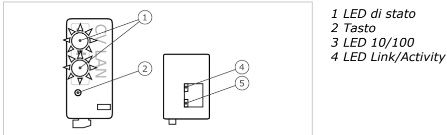
Fig. 2: Panoramica dell'ekey home CV LAN RS-485
