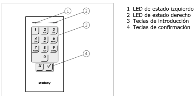
Figura 5: Resumen del teclado numérico
