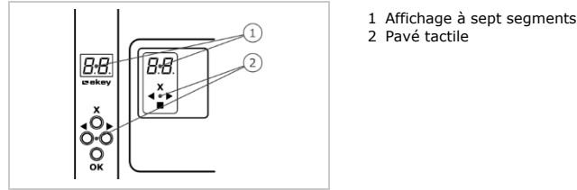
Fig. 6 : Vue d'ensemble de l' ekey home contrôleur en applique et de l' ekey home contrôleur integra
